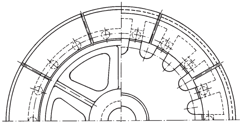
Nabe aus Grauguß ohne Ausfallschlitz | Nabe aus Stahl mit Ausfallschlitz
